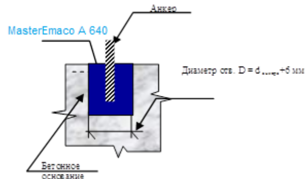
Рисунок 2. Технология крепления анкеров.
